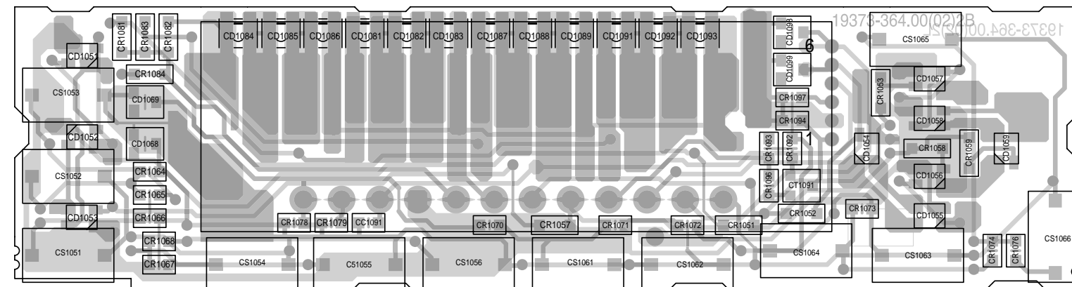
Ansicht von der Bestückungsseite / View of Component Side
